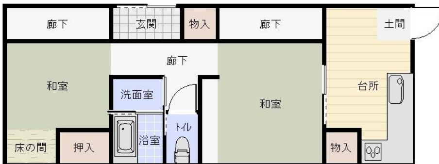
(間取り図)
